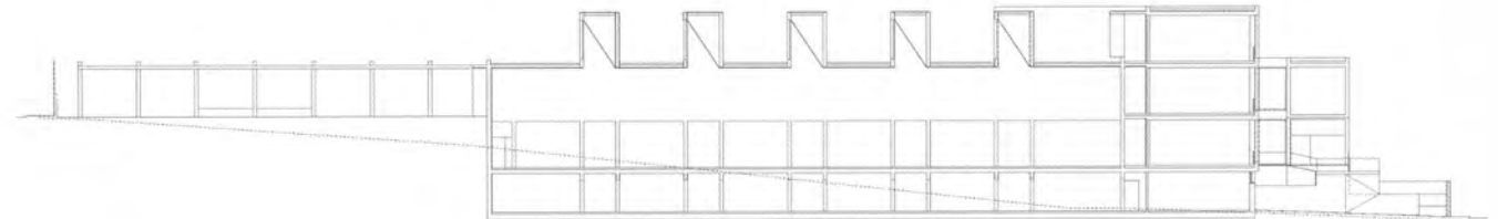
Sección C
