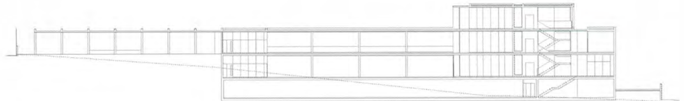
Sección B
